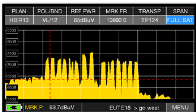
Il satellite puntato non è quello corretto. Nella parte bassa del display compare la seguente informazione: EUTE 16 > GO WEST (muovi la parabola verso Ovest).
