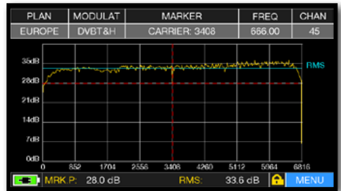
MER vs CARRIER : modalità di visualizzazione "VIS. TYPE: NORMAL" e "PICTURE: CONTOURS".
