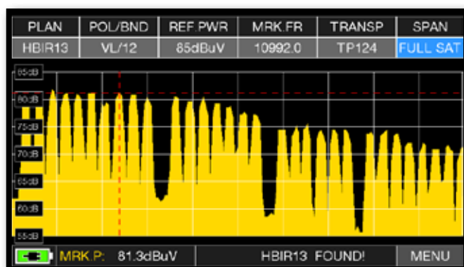
Satellite trovato. Nella parte bassa del display compare la seguente informazione: HBIR13 FOUND ! (il satellite puntato è quello corretto).
