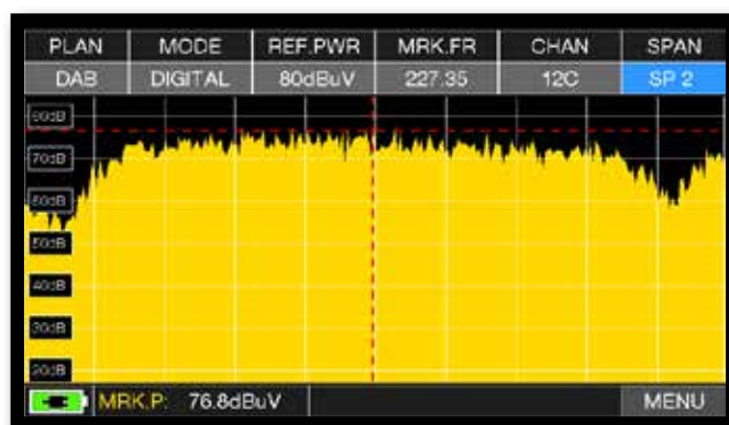
Spettro "DAB" SPAN 2 MHz.
