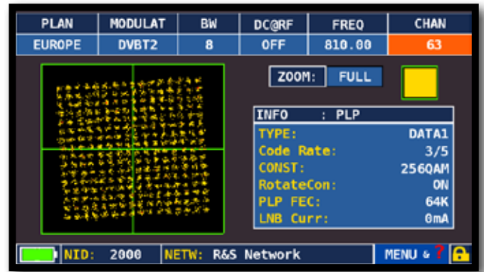
Costellazione DVB-T2
