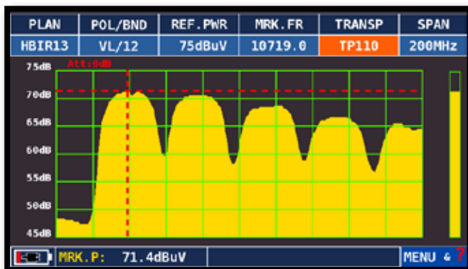
Spettro SAT.
