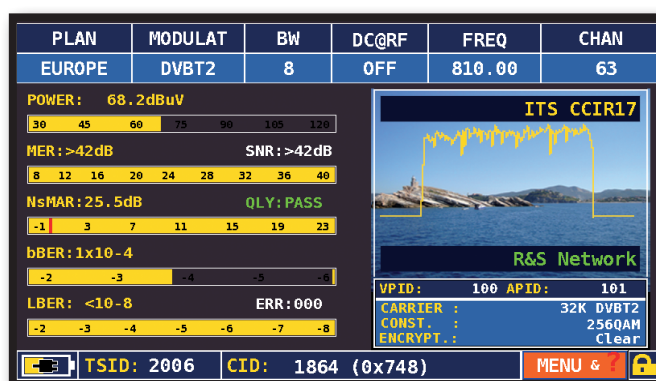
TV Mini spectrum
