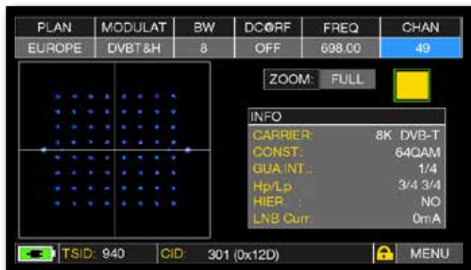
Costellazione DVB-T
